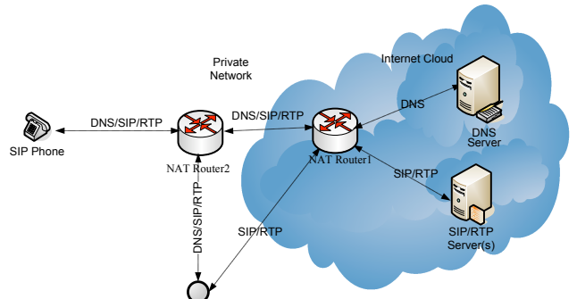
(b) SIP phone behind NATs
